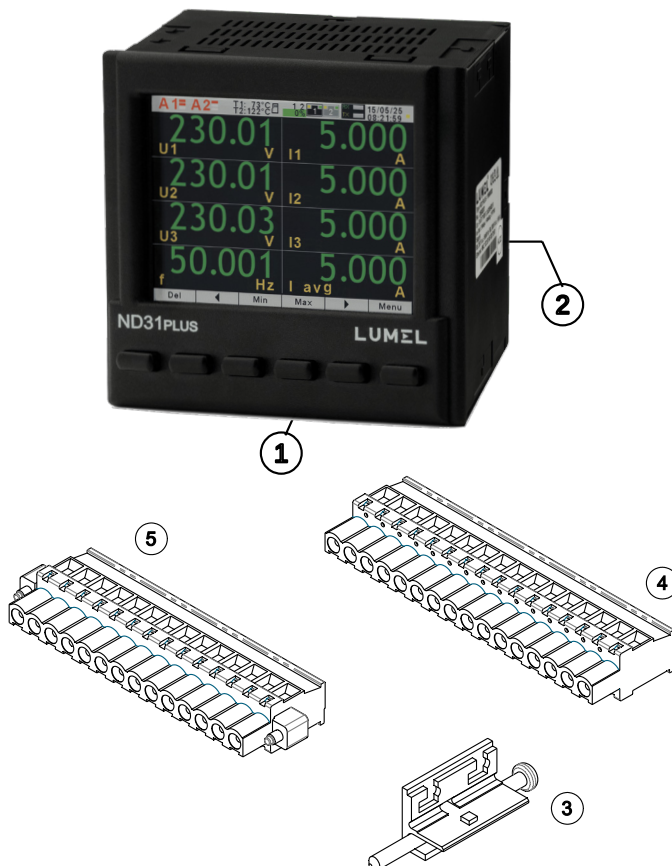
Fig. 1. Meter set
