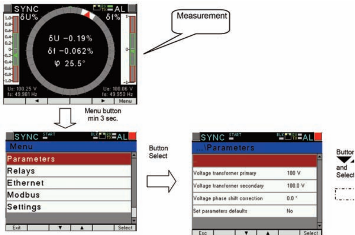
Fig.12, Screens of Parameter group
