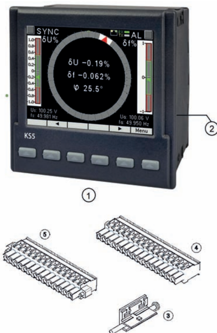
Fig.1, Meter set
