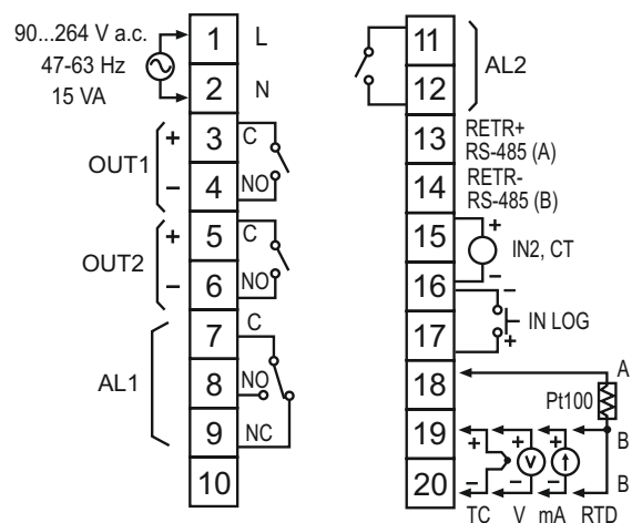
Terminal strip RE41, RE42
