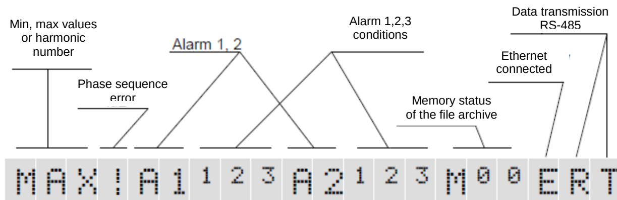
Fig.10. Information bar
