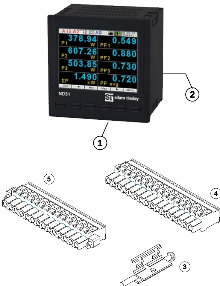
Fig. 1. Meter set
