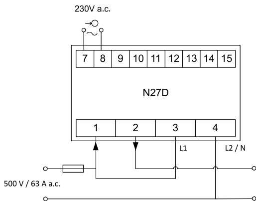
Rys. 2. Połączenia elektryczne miernika N27D
