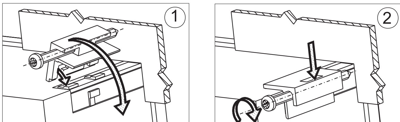
Fig. 1. Meter fixing
