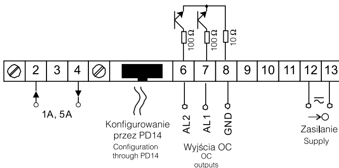
Rys. 4. Połączenia elektryczne miernika N20Z z pomiarem prądu
