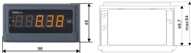
Rys. 2. Gabaryty miernika N20Z i N20ZPLUS
